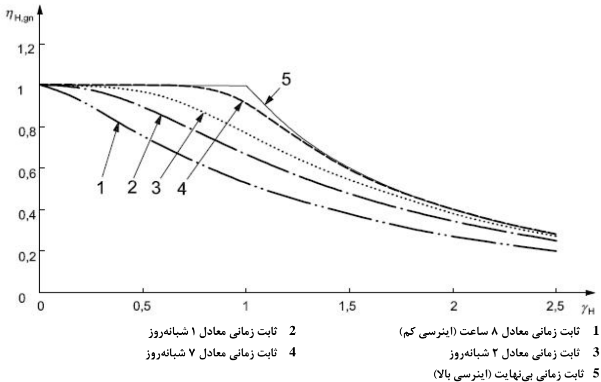
شکل الف-۳- تغییرات ضریب جذب حرارت بر حسب نسبت بالانس حرارت در حالت گرمایش برای ثابت های زمانی مختلف
