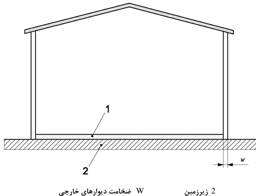
شکل الف-۱۱- نمودار شماتیک کف روی خاک
